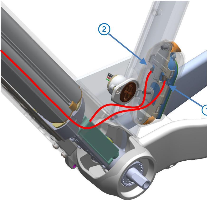
Trou passe câble/inlet cable hole
