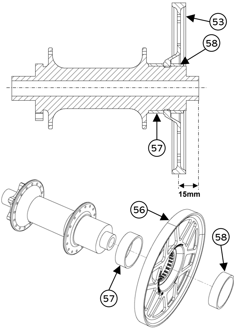
Clutch 150.7 EQ / 160.8 / 160.7
