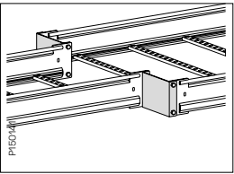
Voidaan myös keskittää hyllyjä.
