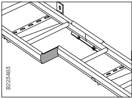
Kavennuskappale 31 saadaan muutettua tikashyllyjen leveyksiä.
