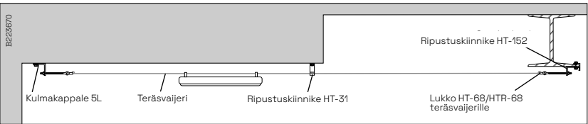
Teräsvaijeri asennettuna kattoon.
