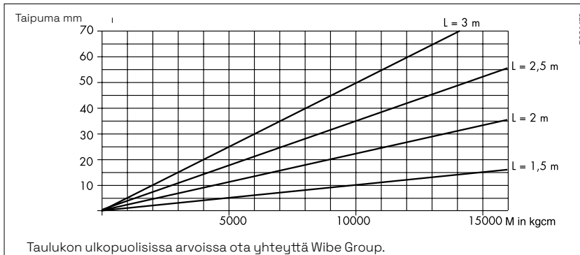
M = \sum F \times A Huomio myös seinäkannake 50 maksimi kuormat asennus-/ ankkurikisko asennuksissa (katso seinäkannake 50L, 50 ja 50F sivut).
