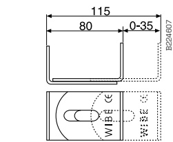
Kulmakappale 5L säädettävyyys
