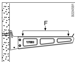
Seinäkannake 50i asennuksessa seinään käytetään kiila-ankkuri M8. Murtokuorma - Katso taulukko.
