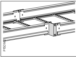
Kavennuskappale 20C saadaan muutettua tikashyllyjen leveyksiä.
