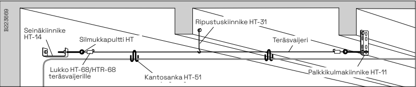
Teräsvaijeri asennettuna kattopalkeista.
