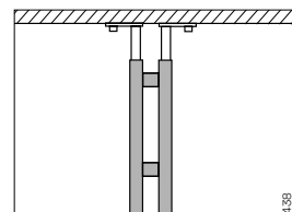
Kattokannake 20F voidaan asentaa lattiaan ja käyttää kattokannaketta 2 kattoon asennettavana kiinnikkeenä.
