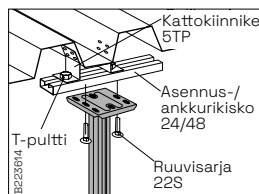
Esim. peltikattoasennuksissa asenna kattokannake 20 kuvan mukaisesti.
