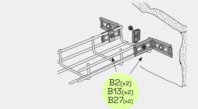
Endefeste mot vegg
