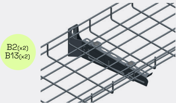
Montering på 50i Konsoll
