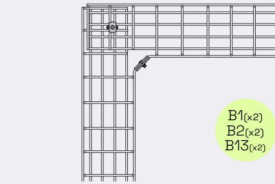
90° avvinkling bredde 522-622 mm
