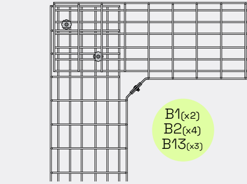
Avvinkling (hvilken som helst vinkel)
