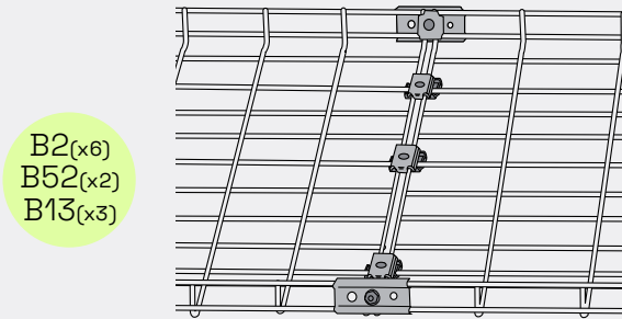
Skjøting nettrenne bredde 522-622 mm
