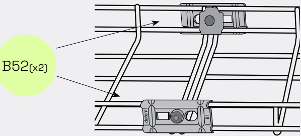
Jatko lankahylly Leveys 422 mm
