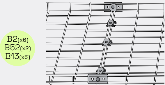
Jatko lankahylly Leveys 522-622 mm
