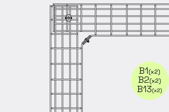
90° Kulma Leveys 522-622 mm
