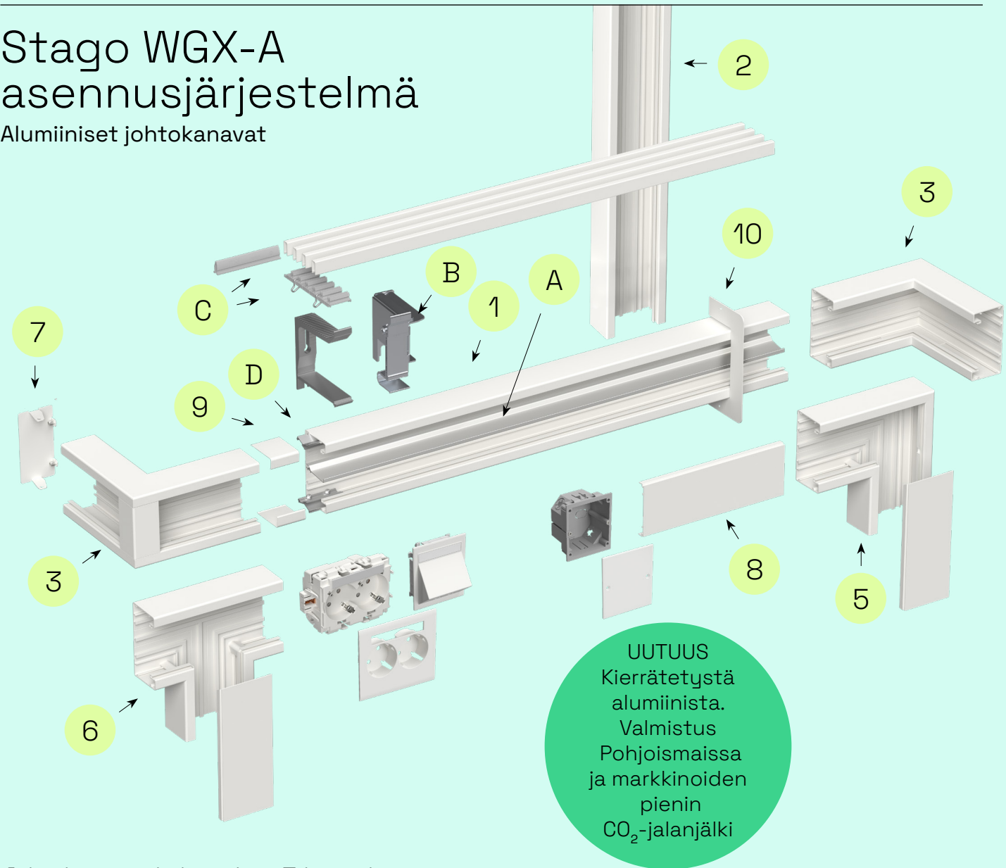
Johtokanavat, kulmat, L- ja T-kappaleet
