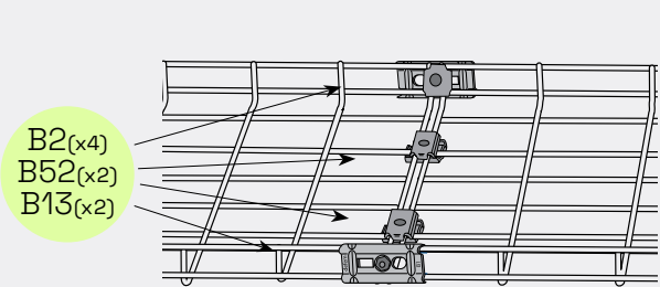
Jatko lankahylly Leveys 422 mm
