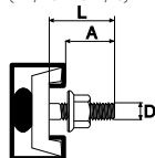
T-bolt 26U/M8 T-bolt 26U/M10 (til P/A-skinne 24/48)
