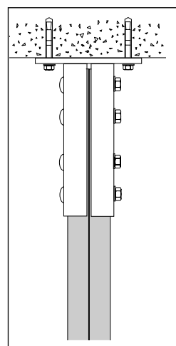
Loftfæste 520 kan monteres som et loft- eller gulvfæste.
