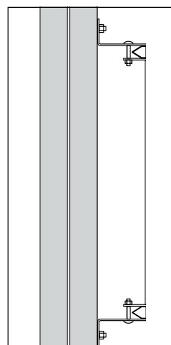
Kabelstige kan monteret vertikalt eller horisontalt på pendel/ankerskinne 24/20 med vægkonsol 11/25 eller 11/75 og T-bolte.
