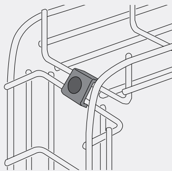
Vertikal avvinkling
