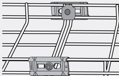
Skarvning trådstege bredd 422 mm
