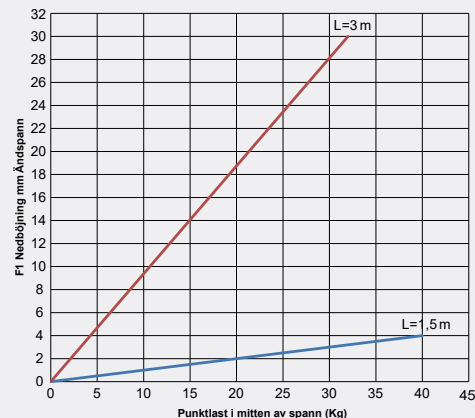
Armaturskena W70/70-200
