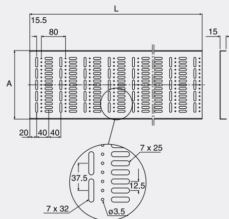
Armaturskena W70-50
