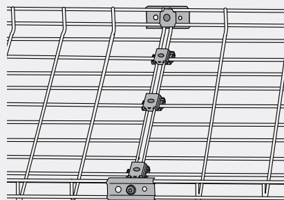
Vertikal avvinkling
