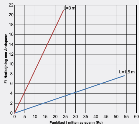
Armaturskena W70/70-200
