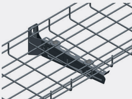
Montage på Konsol 50i
