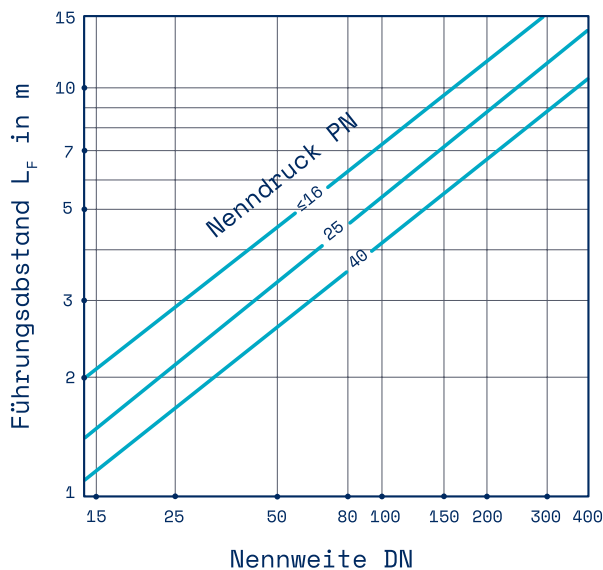
Bild4: Empfohlene Abstände für Rohrführung bei axial kompensierten Leitungen
