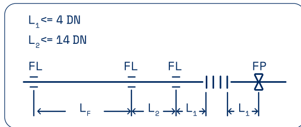
Bild 3: Führungsabstände von Rohrleitungen mit Axial-Kompensatoren
