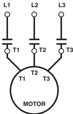
3 FASE
